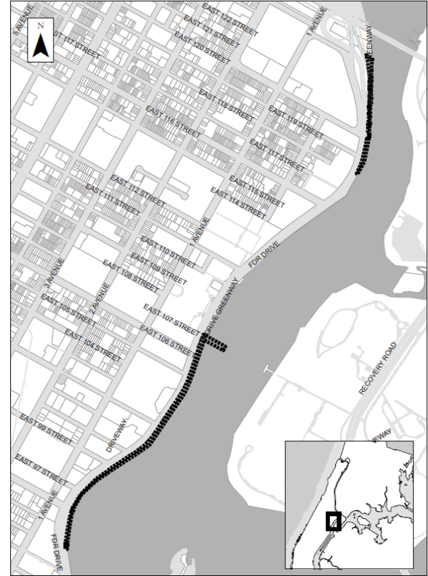
Context Map
